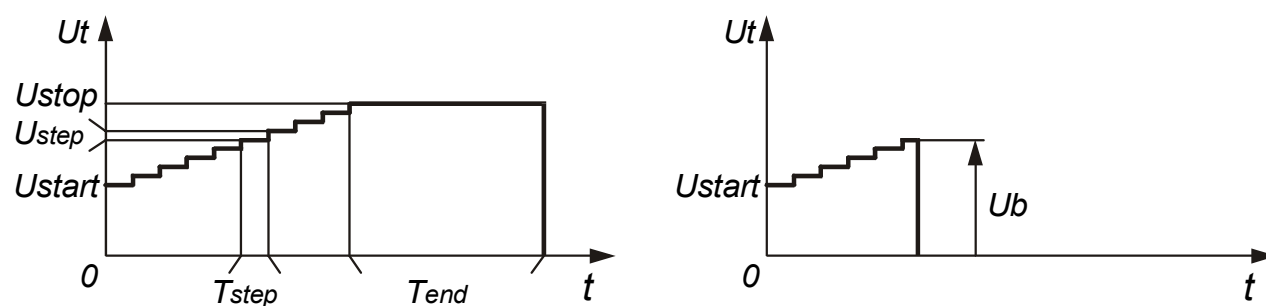
Рис. 17 Испытательное напряжение без пробоя (слева) и с пробоем (справа)
