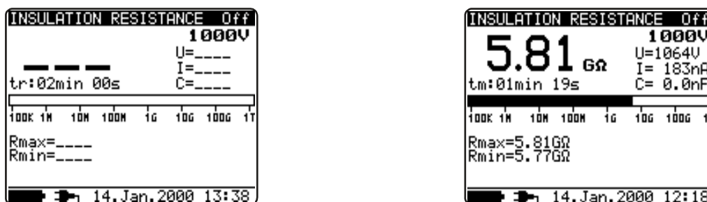
Рис. 9 Состояния дисплея в функции измерения сопротивления изоляции
