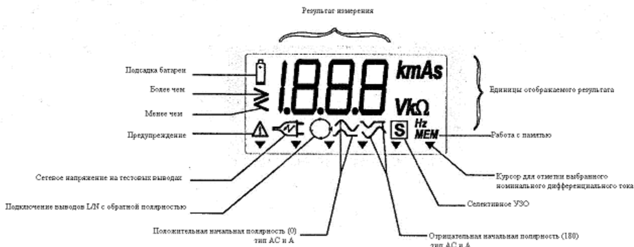
Рис. 4 Сегменты дисплея
