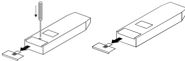
Рис.5. Вскрытие отсека элементов питания.
