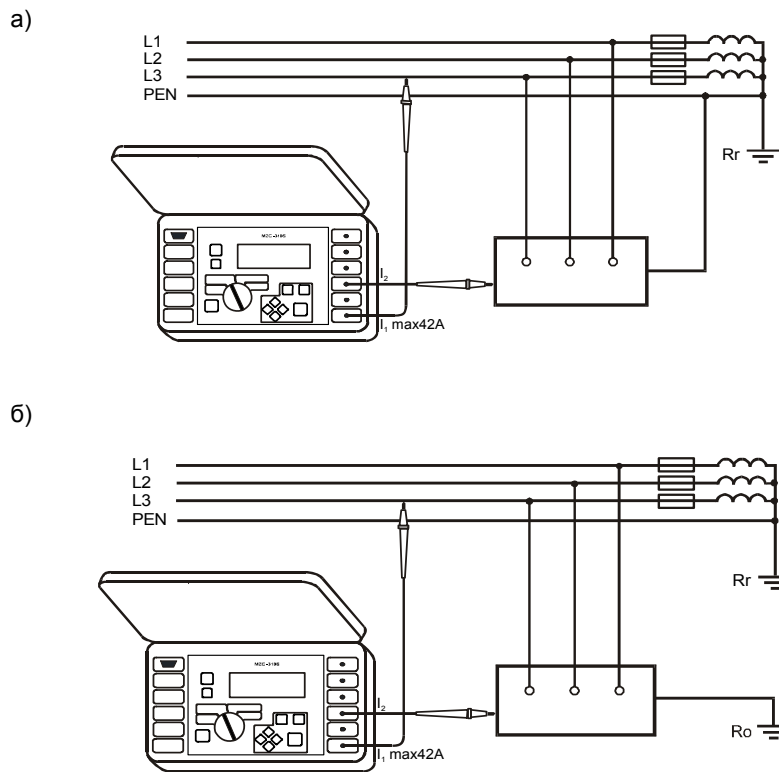
Рис.16. Проверка эффективности защиты корпуса электроустановки двухполюрным методом в случае: а) сети TN, б) сети TT
