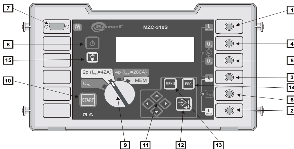
Рис.1. Расположение гнезд и клавиш в измерителе MZC-310S (передняя панель)
