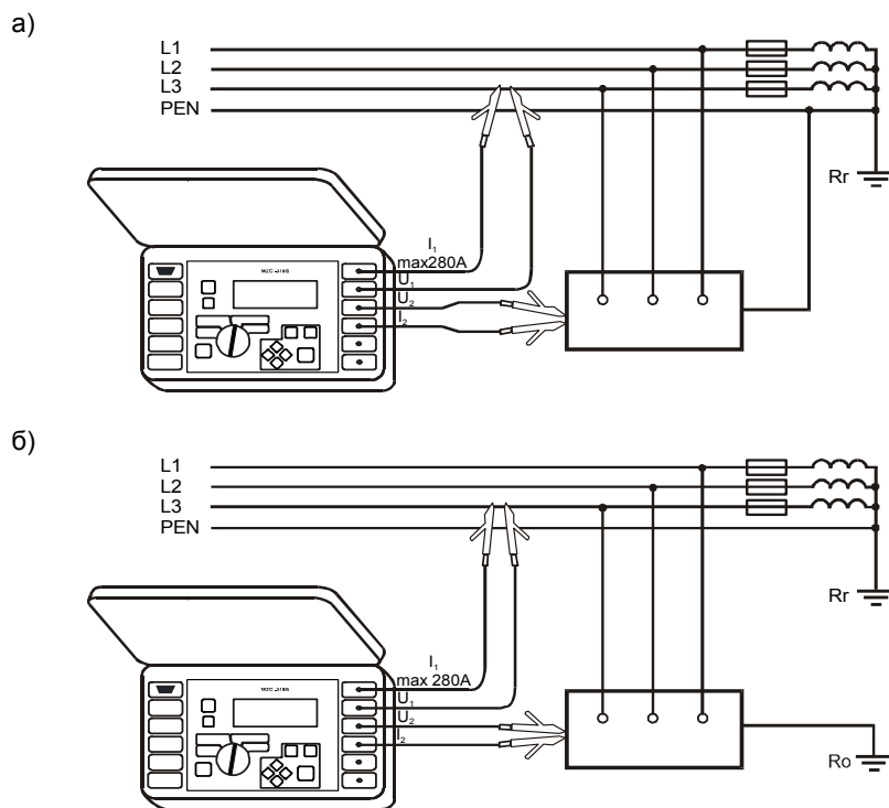
Рис.17. Проверка эффективности защиты корпуса электроустановки четырёхполюрным методом в случае: а) сети TN, б) сети TT
