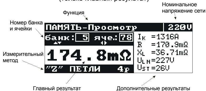
Рис.4. Вид экрана в режиме измерения полного сопротивления петли короткого замыкания (только главный результат)
