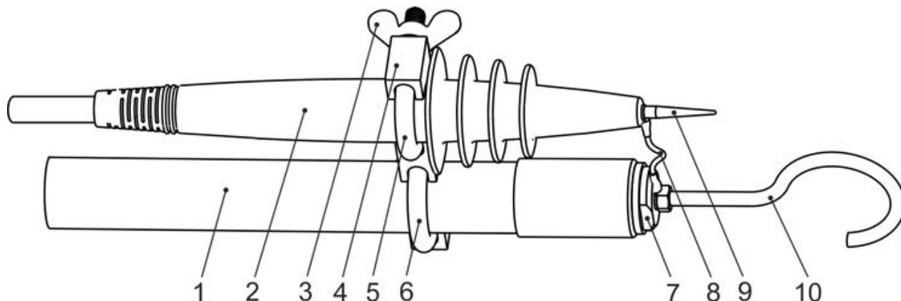
Рисунок 6 – крепление щупа измерительного кабеля к штанге оперативной, где: 1 – штанга оперативная ШО-35 (поставляется по отдельному заказу);
