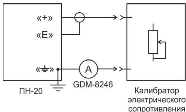
Рисунок 12 – Измерение сопротивления изоляции и силы тока
