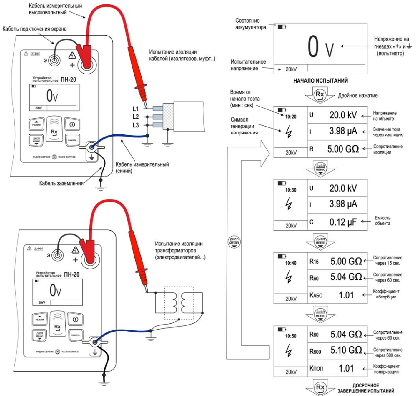
Рисунок 7 – Схема подключения и показания индикатора при испытаниях изоляции
