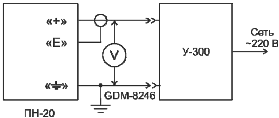
Рисунок 13 – Измерение напряжения переменного тока
