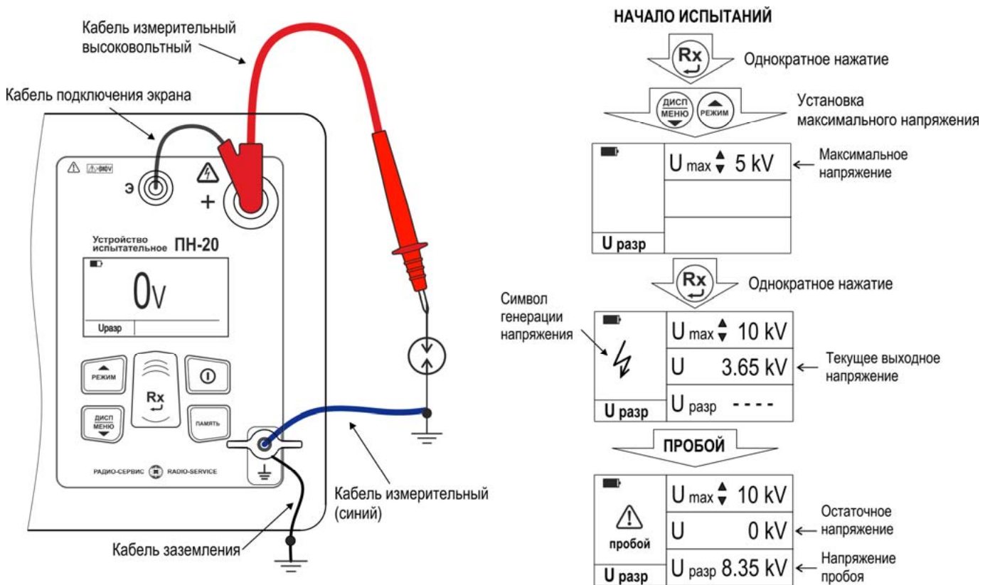
Рисунок 8 – Проверка напряжения пробоя разрядников
